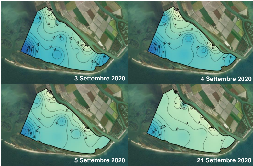
Figura 16. Distribuzione dei valori di salinità in superficie nel mese di settembre 2020 a seguito del completamento del manufatto idraulico.
