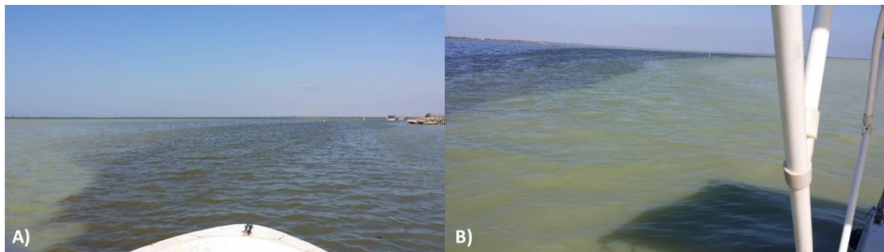
Figura 8. Stazione Conca (A) e stazione VS2 (B) durante l'anossia di fine luglio 2015.
