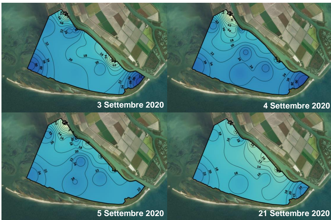
Figura 17. Distribuzione dei valori di salinità sul fondo nel mese di settembre 2020 a seguito del completamento del manufatto idraulico.
